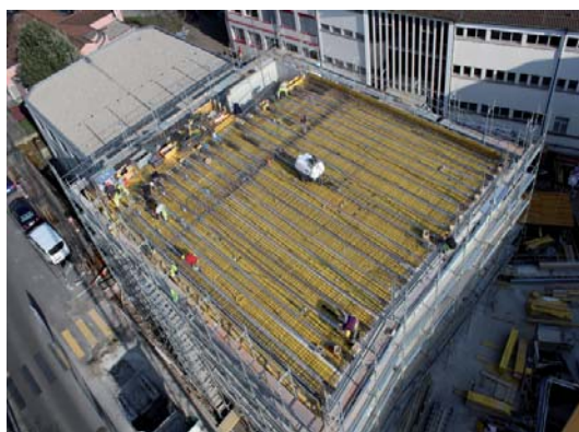
Dalle précontrainte
